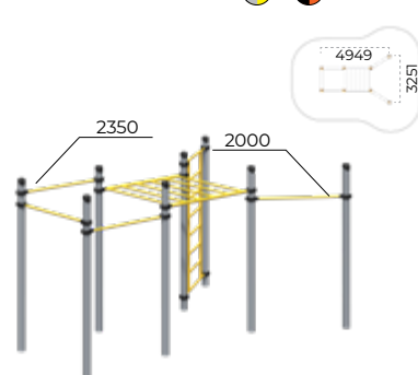
Оборудование спортивное Romana 501.58.01
