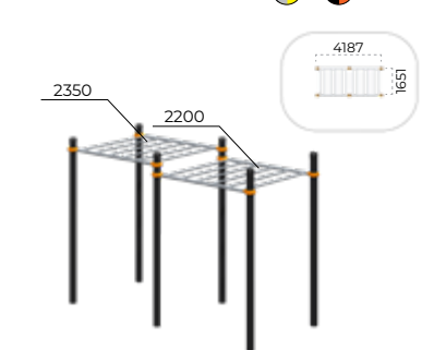
Рукоход 2-уровневый Romana 501.23.01
