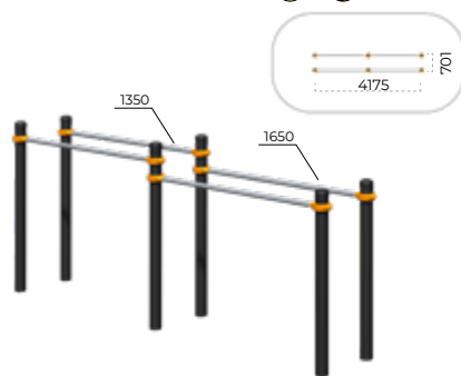
Брусья разновысотные Romana 501.18.01
