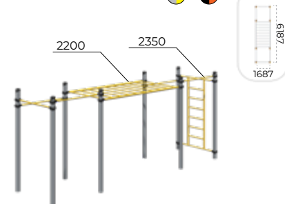
Комплекс с рукоходом Romana 501.16.01
