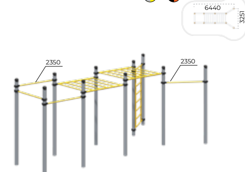
Оборудование спортивное Romana 501.54.01
