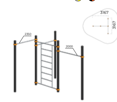
Оборудование спортивное Romana 501.37.01
