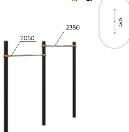
Турник сдвоенный Romana 501.26.01
